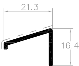
L50804 pingadeira tradicional
