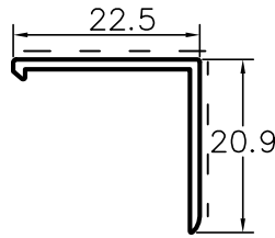
L50805 pingadeira tradicional
