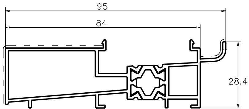
L53705 soleira
