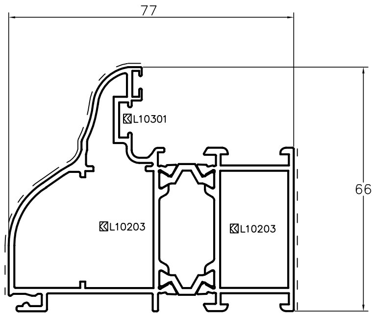
L53054 aro decorativo c/ remate
