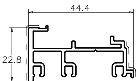
L53841 remate inferior
