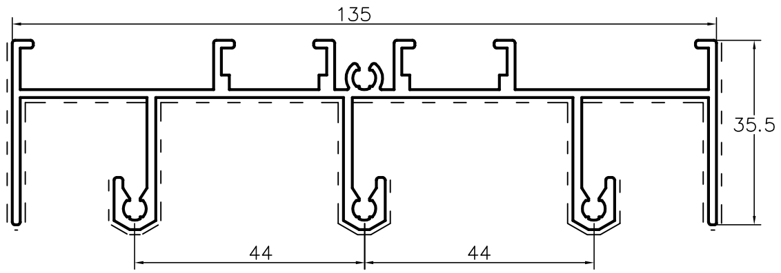
L62141 padieira tri-raíl
