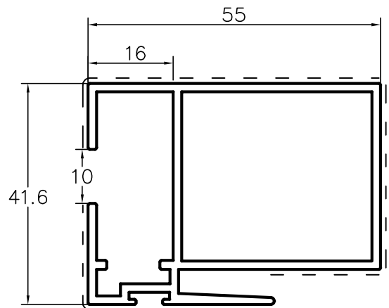
L62471 central invertido 3 folhas
