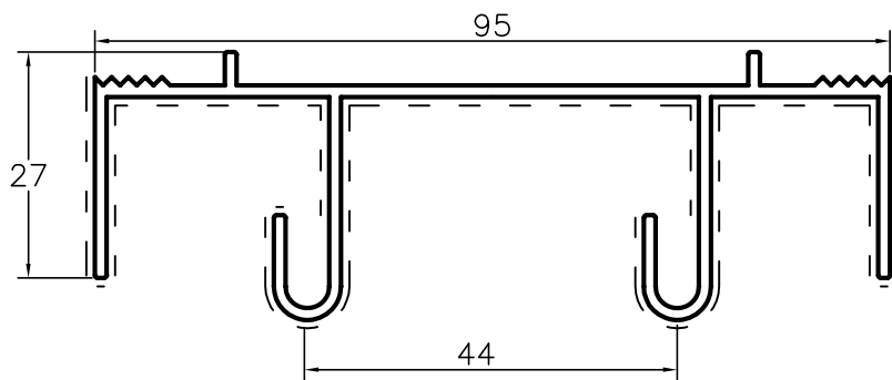
L62101 padieira tradicional
