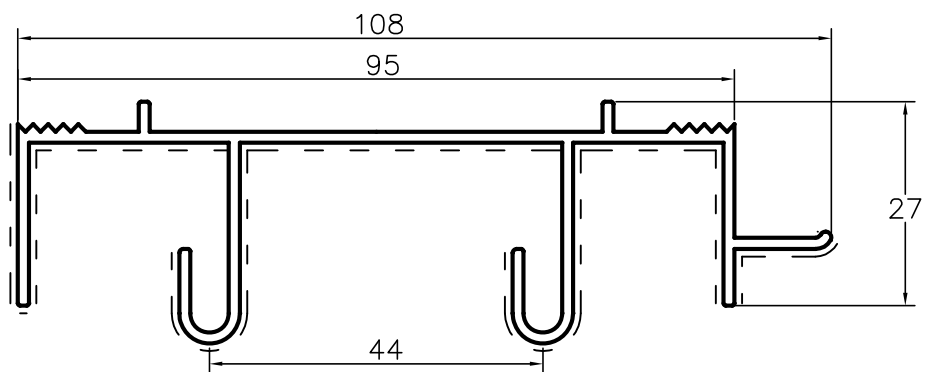
L62131 padieira tradicional
