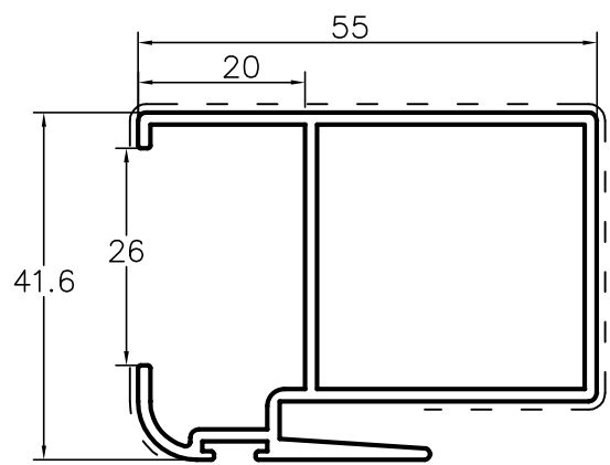
L62472 central invertido 3 folhas
