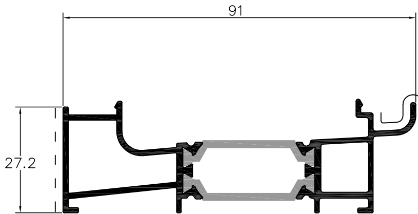
L56701 soleira
