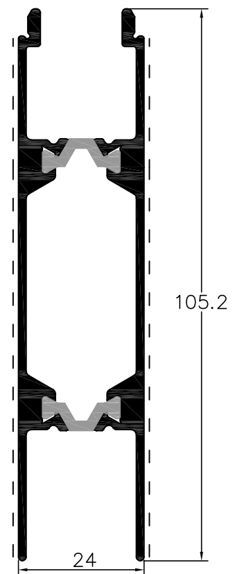
L53821 régua
